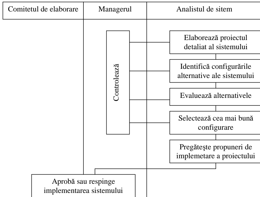
Fig. 2. Faza de proiectare a sistemului informațional
